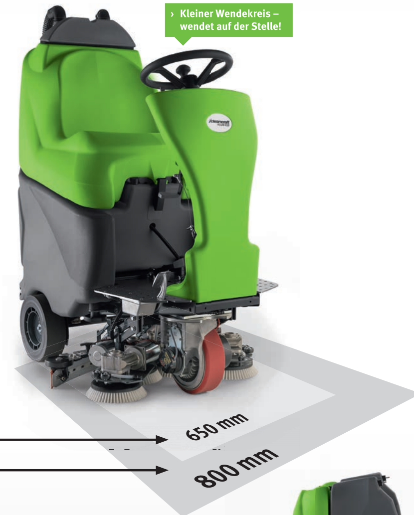
Vier kleine Scheibenbürsten, mit direkt dahinter liegender Absaugleiste, ermöglichen eine kurze Bauform und einen sehr kleinen Wendekreis
