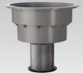
Schutz-Einlage mit integriertem Schwimmer verhindert beim Nasssaugen das Eindringen von Flüssigkeit in die Filter oder Saugmotoren
